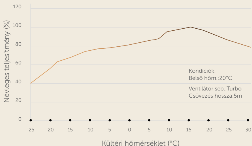
2,5 és 3,5 kW-os Comfort X fűtési teljesítménye különböző külső hőmérsékletek mellett
